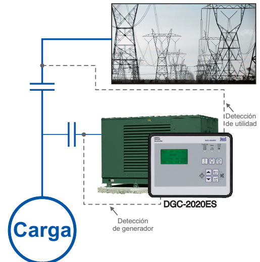
Figura 1: Diagrama de conexiones de DGC-2020ES típicas
